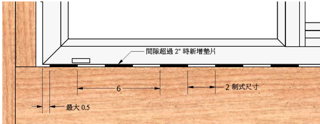
框檻示意圖
