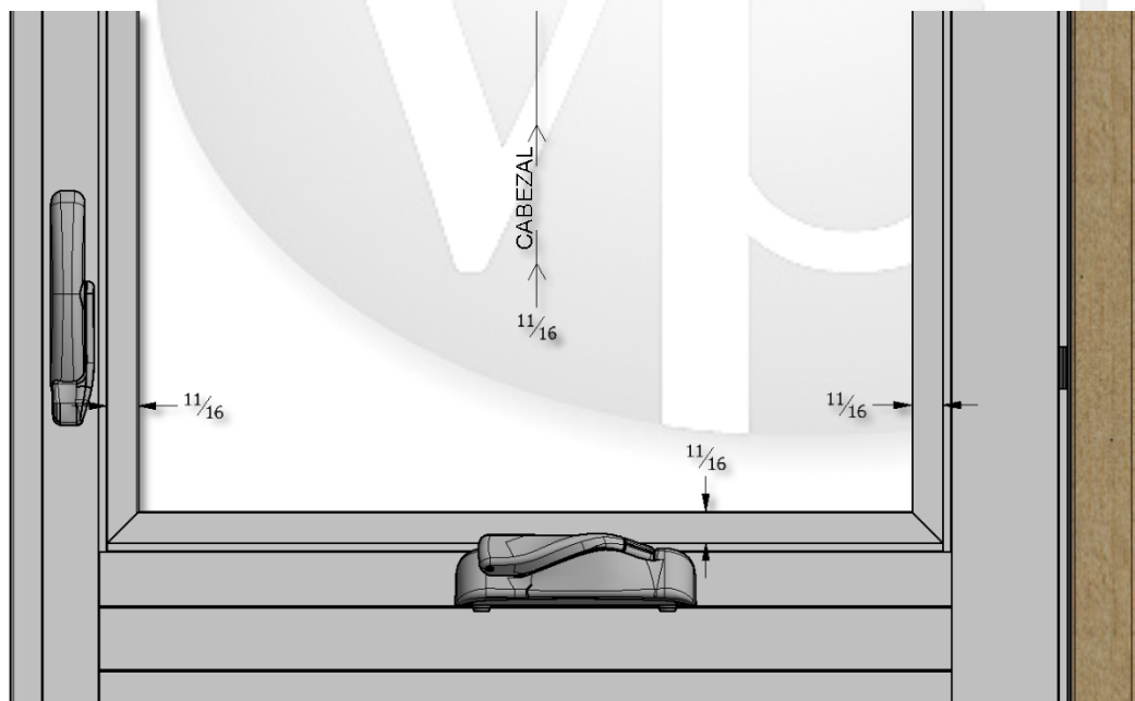
Figura 13 Vista de la profundidad
