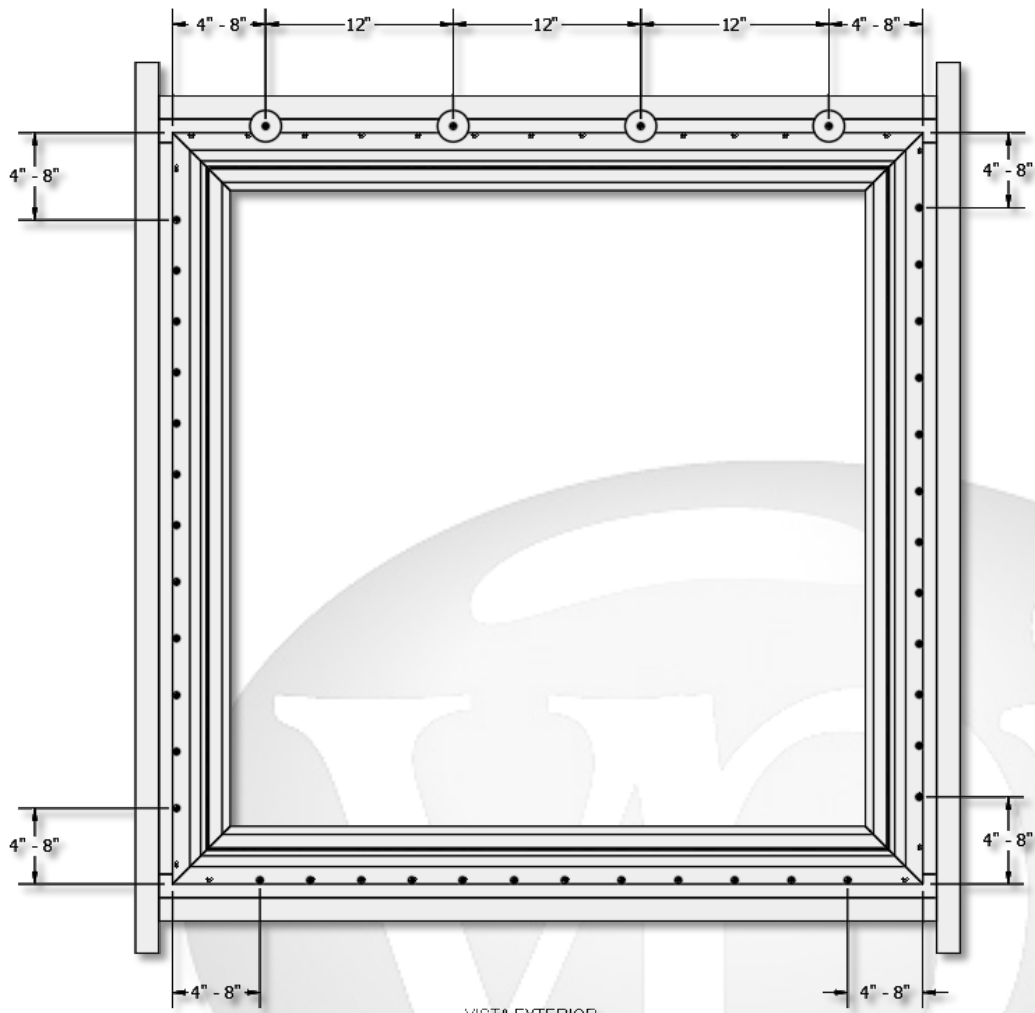
VISTA EXTERIOR ESCALA 1/8
