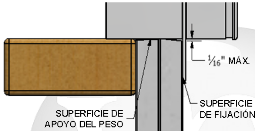
Figura 2 Estado aceptable (planitud)
