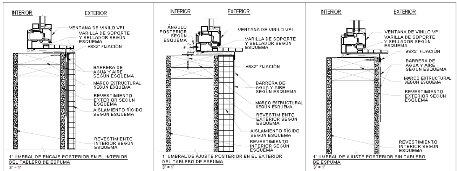
C) DETALLES DE LA ALETA CLAVADA A 1.375 IN (3.49 CM) DE ENCAJE POSTERIOR DE LA CARA EXTERIOR
