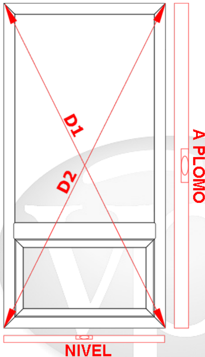
Figura 7 Vista de cuadratura del marco
