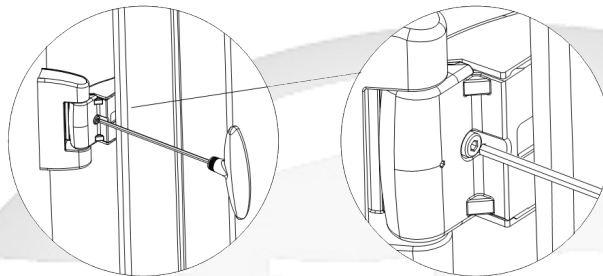
Рис. 23: Регулировочный болт
